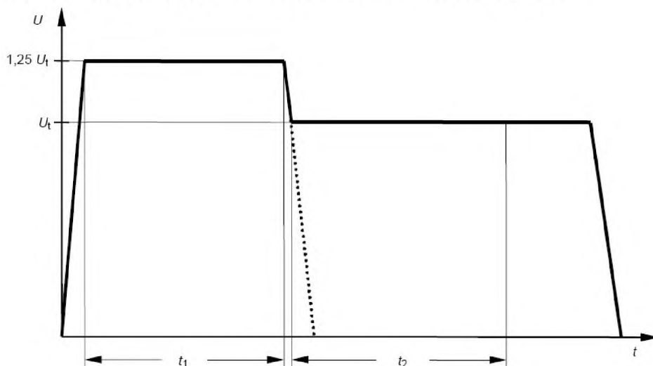
Рисунок 1 – Испытательное напряжение
