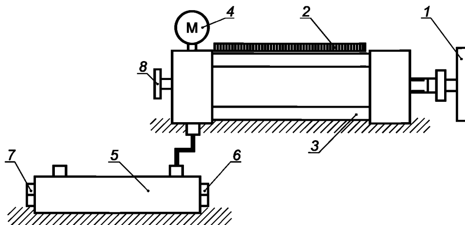
1 — маховик; 2 — измерительная линейка; 3 — гидроцилиндр; 4 — манометр; 5 — пробоборборник; 6 — входной вентиль пробоборборника; 7 — выходной вентиль пробоборборника; 8 — вентиль гидравлического пресса
