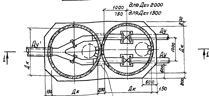
План КД-1
