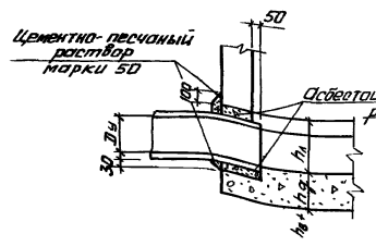
Заделка труб в непросадочных сухих грунтах
