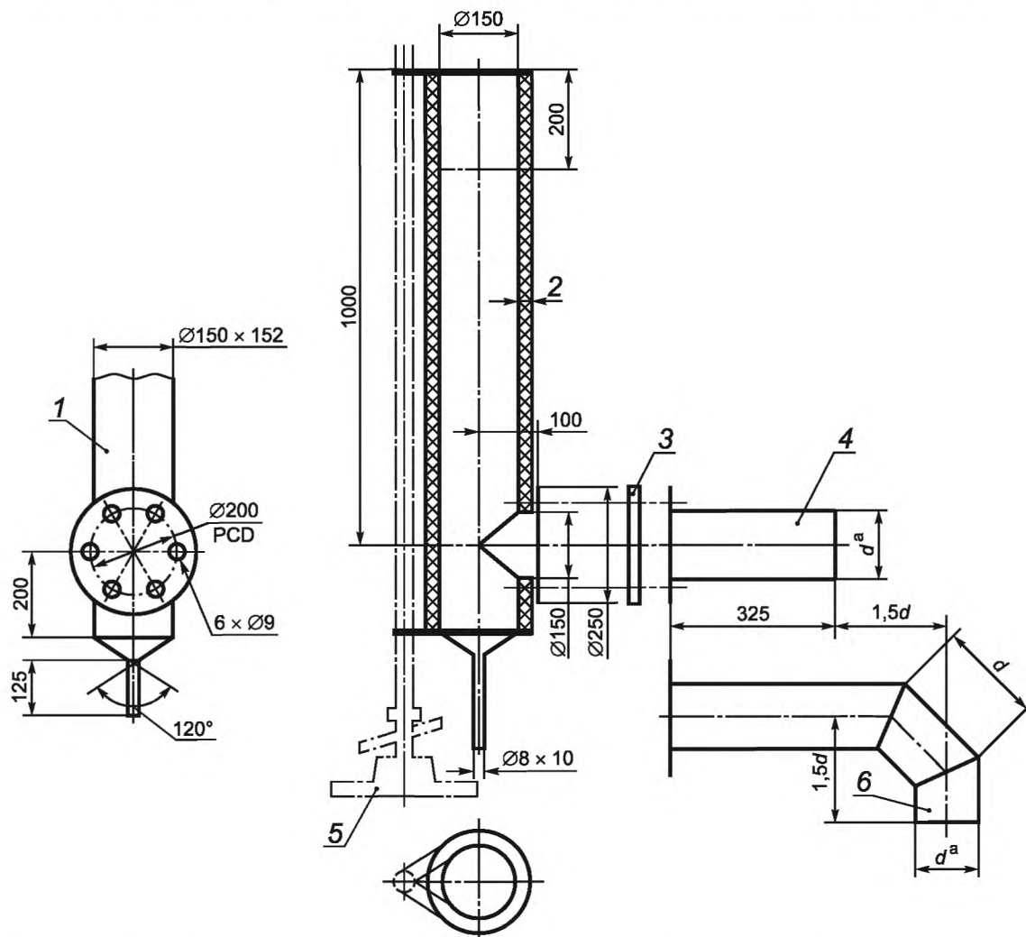
1 — труба дымохода из нержавеющей стали; 2 — теплоизоляция (стекловолочно плотностью 64 кг/м 3 ); 3 — прокладка; 4 — соединительная труба из нержавеющей стали; 5 — опорная стойка; 6 — соединительная труба из нержавеющей стали
