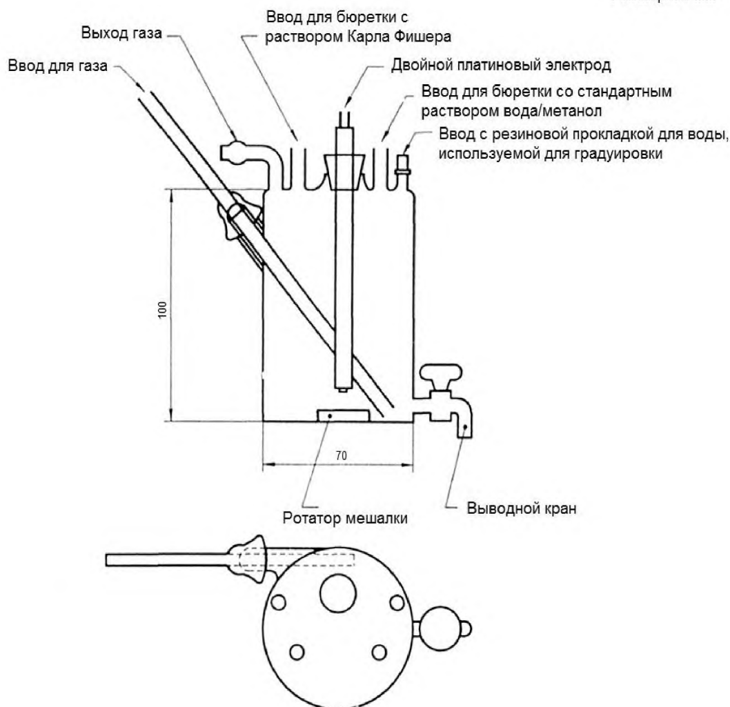
Рисунок 5 - Поглотительная ячейка
