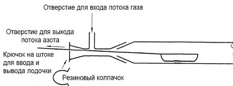
Рисунок 2 - Осушительная трубка
