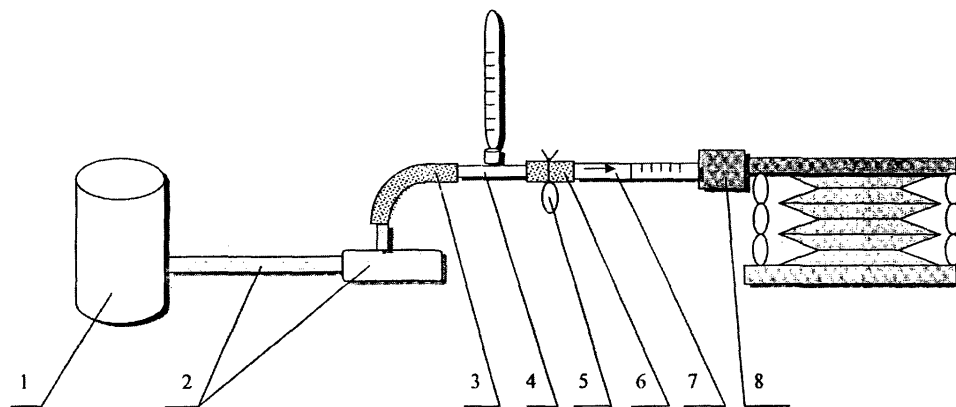
Схема отбора проб промышленных выбросов из газохода
