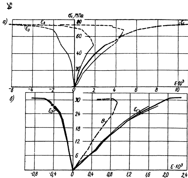
Рис.27. Напряжения-деформации тяжелого крупнозернистого бетона - \bar{R} = 44 \text{ МПа}
