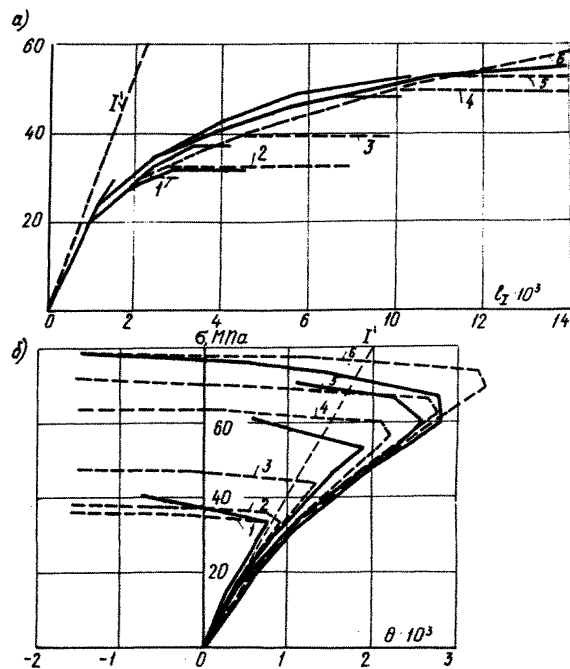
Рис.28. Экспериментальные (—) и теоретические (---) данные по напряжениям-деформациям - \sigma_1 + \epsilon_2 - (а) и \sigma + \theta - (б) для тяжелого крупнозернистого бетона - \bar{R} = 48,6 \text{ МПа}
