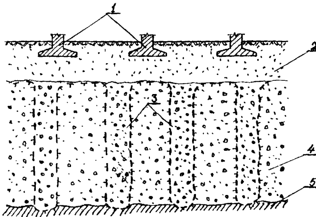
Рис.1. Схема устройства локально оттаянного основания при передаче нагрузок через распределительный слой:
