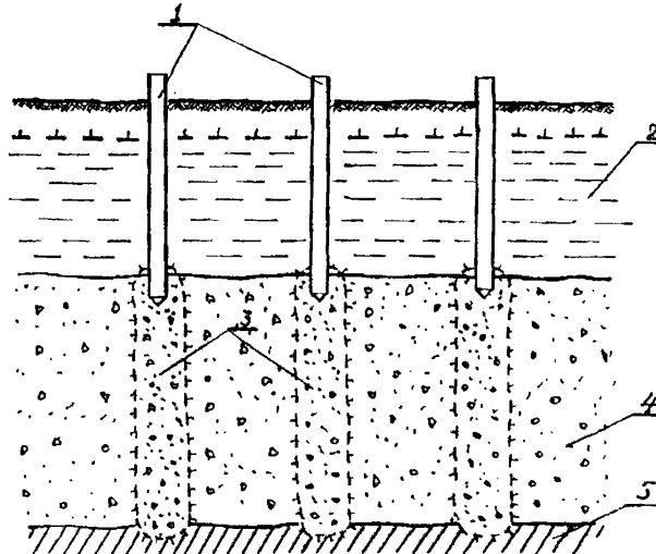
Рис.2. Схема устройства основания при опирании свай-стоек на локально оттаявшие зоны грунта:
