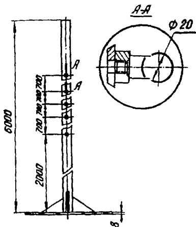
Рис.20. Поверхностная марка
