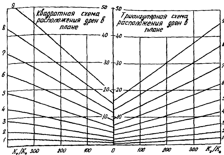
Рис. 6. Графики для определения степени консолидации Q_z слабых грунтов с комбинированными дренами при мгновенном приложении уплотняющей нагрузки (а) и для определения параметра d_e^2 \cdot F(\nu) (б)
