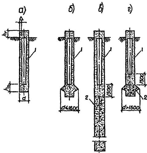
Рис. 1. Типы набивных полых свай: I - малоподвижная бетонная смесь; 2 - литая бетонная смесь или малоподвижная бетонная смесь, уплотненная глубинными вибраторами
