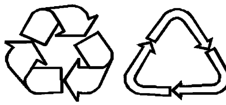
а, б— петля Мёбиуса
