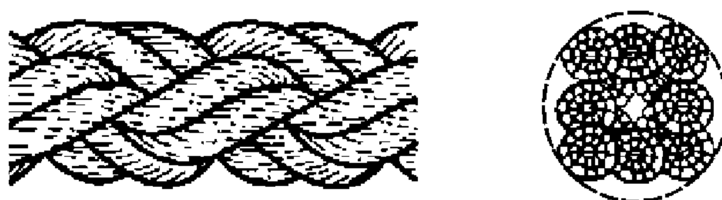
Рисунок 2 — Конфигурация 4-рядного крученого каната (тип В)
