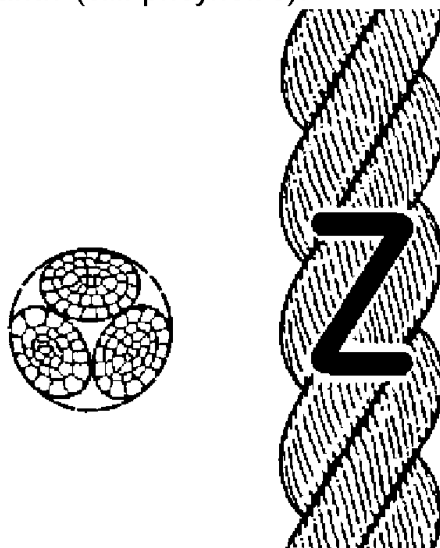
Рисунок 1 — Конфигурация 3-рядного крученого каната (тип А)
