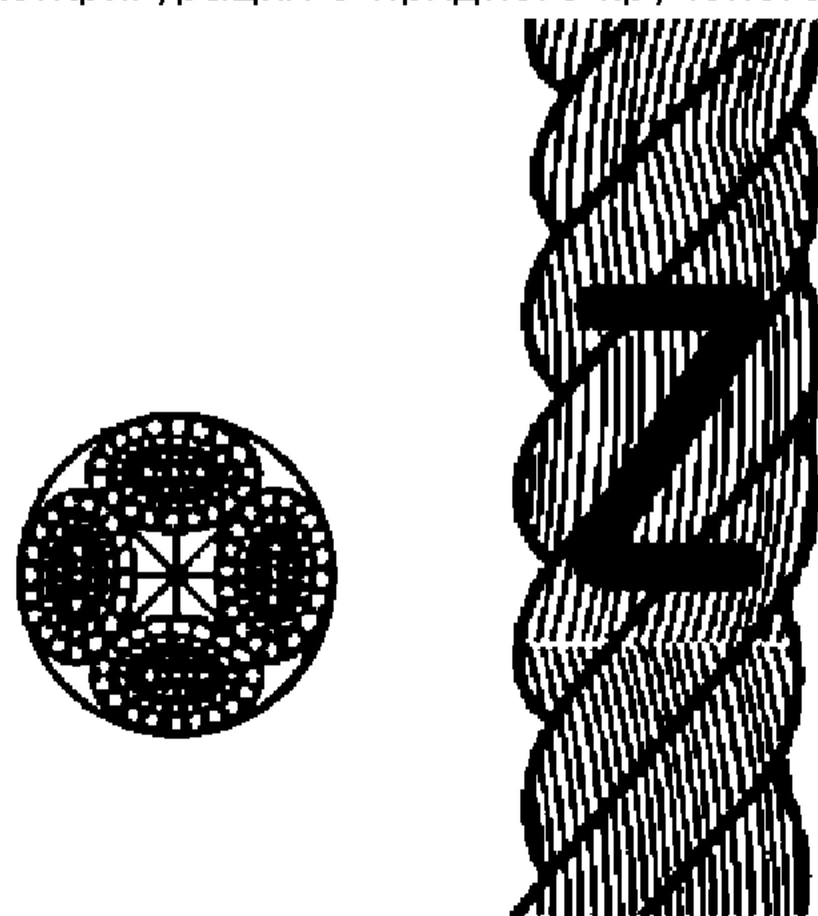
Рисунок 1 — Конфигурация 3-рядного крученого каната (тип А)
