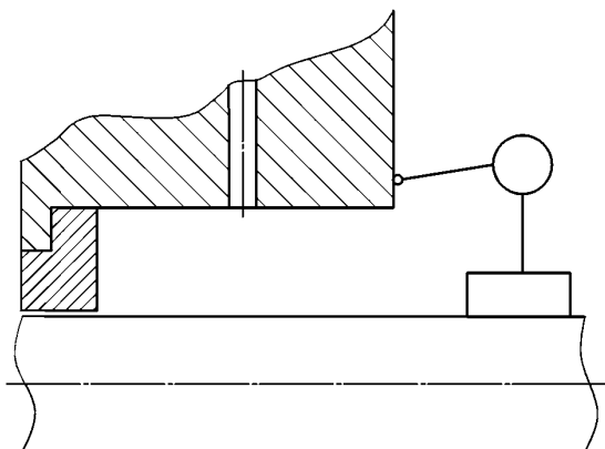
Рисунок 15 — Торцовое биение камеры уплотнения
