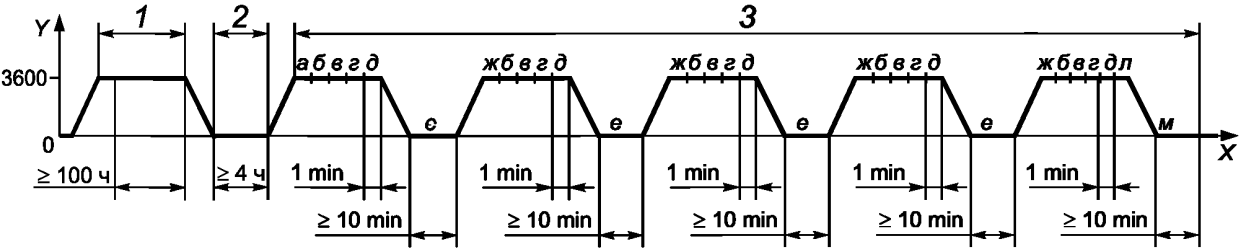
X — время; Y — скорость (об/мин); 1 — фаза динамической проверки; 2 — фаза статической проверки; 3 — фаза циклической проверки;
