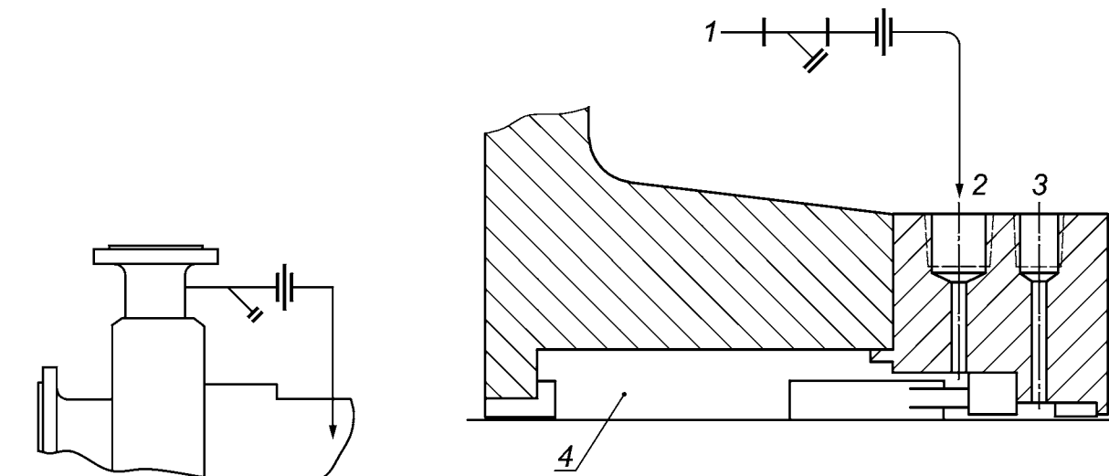
а) Трубопровод и схема измерительного прибора б) Детали камеры уплотнения
