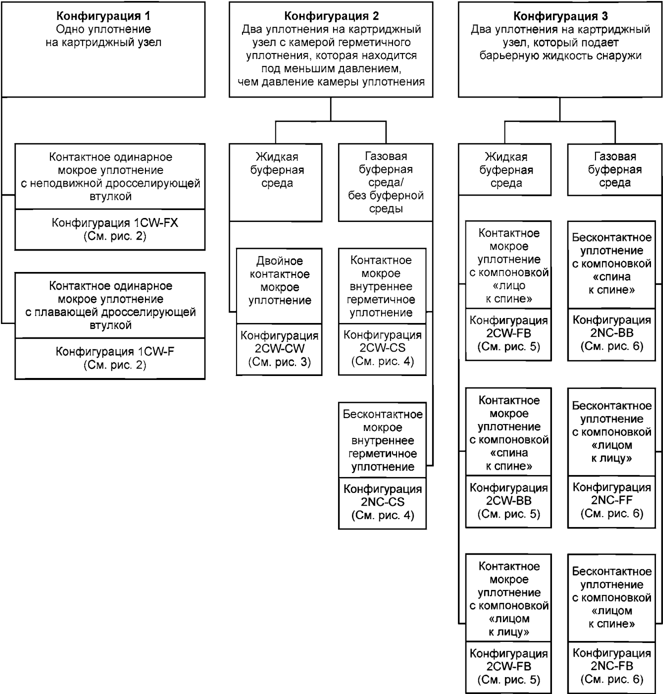
Рисунок 1 — Конфигурация уплотнения
