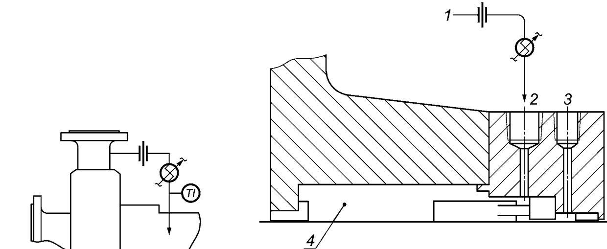
а) Трубопровод и схема измерительного прибора б) Детали камеры уплотнения
