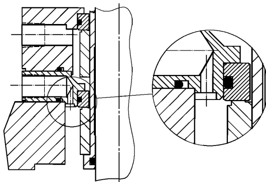
Рисунок 17 — Камера уплотнения/фланец корпуса уплотнения вертикальных насосов
