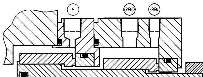
в) конфигурация «сдвоенное уплотнение с подачей буферной жидкости без давления (тандем)», 3NC-FB, бесконтактные уплотнения
