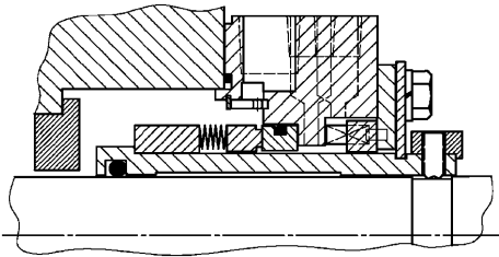
а) Стандартное (вращающийся узел сифона)
