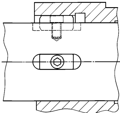
Рисунок 24 — Крепление шпонки к валу
