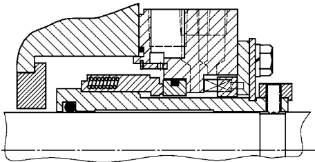
а) Стандартное (вращающийся упругий элемент)
