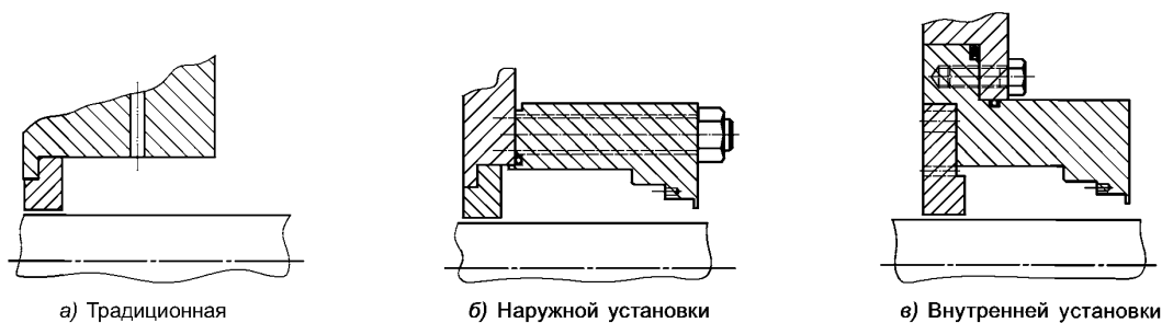
Рисунок 12 — Типы камер уплотнения
