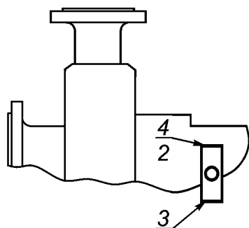
а) Трубопровод и схема измерительного прибора
