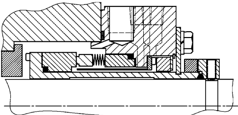
а) Стандартное (неподвижный узел сифона)
