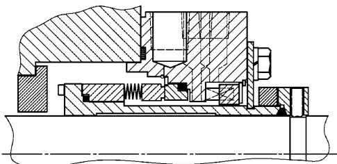
б) Альтернативное (вращающийся узел сифона)
