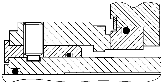
Рисунок 25 — Устройство вспомогательной втулки
