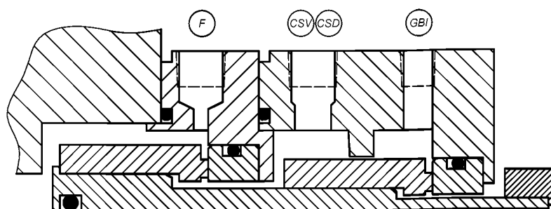
а) 2CW-CS, контактное жидкостное резервное внутреннее уплотнение
