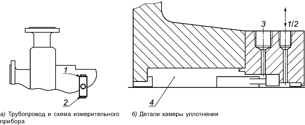
Рисунок Ж.18 — Схема 54 промывки стандартного уплотнения
