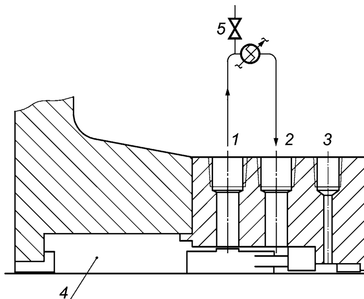
б) Детали камеры уплотнения
