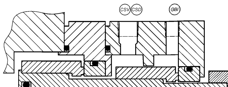
б) 2NC-CS, бесконтактное резервное внутреннее уплотнение
