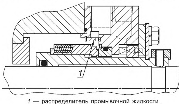
Рисунок 22 — Система распределения промывочной жидкости уплотнения
