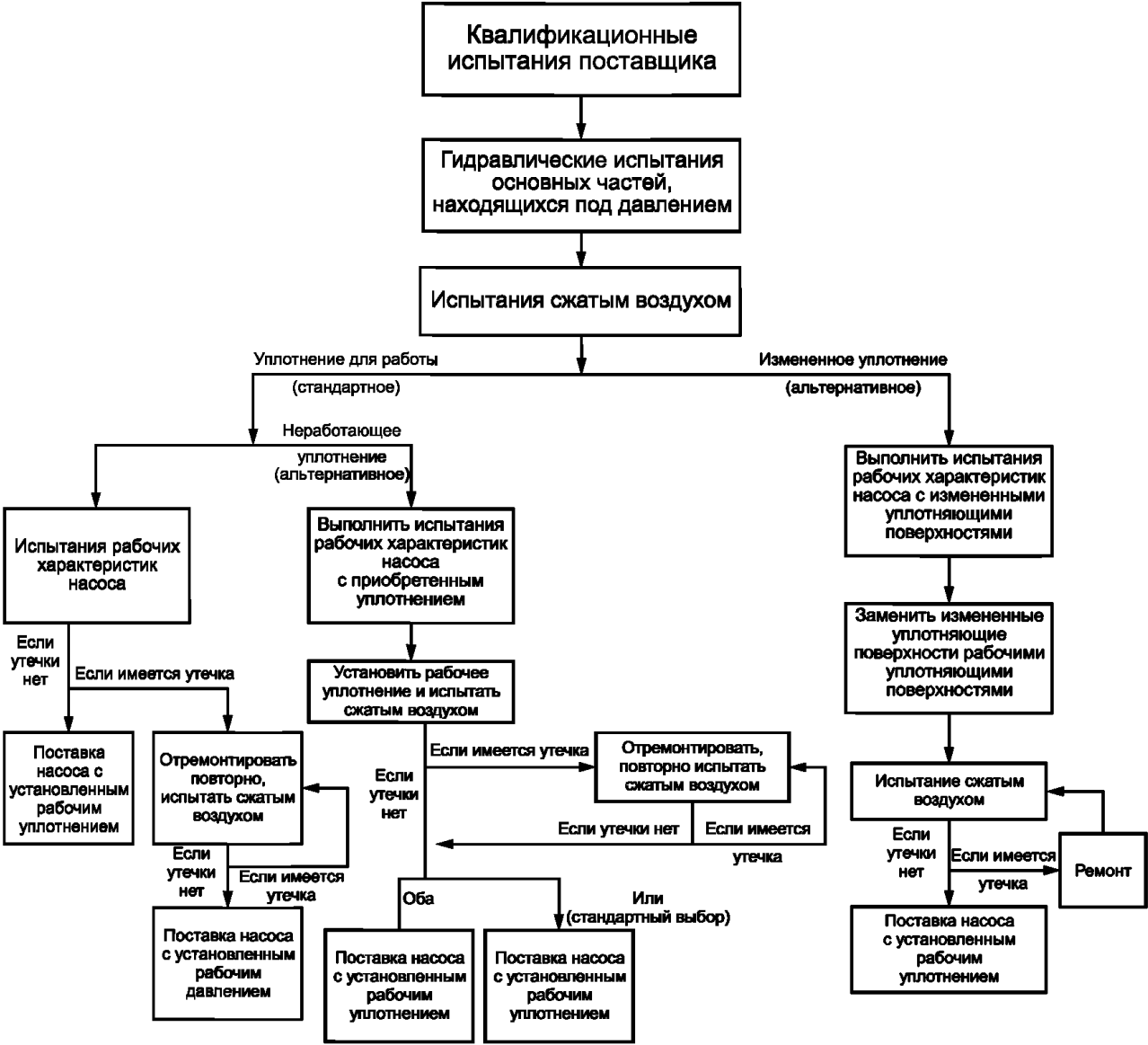
Рисунок 27 — Последовательность действий при проведении испытаний
