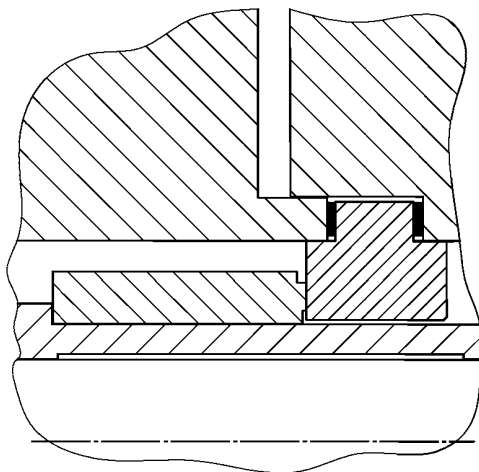
Рисунок 21 — Фиксация поверхностей
