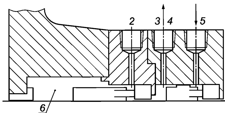
б) Детали камеры уплотнения
