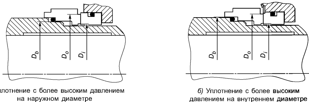
Рисунок 10 — Точки измерений соотношения баланса
