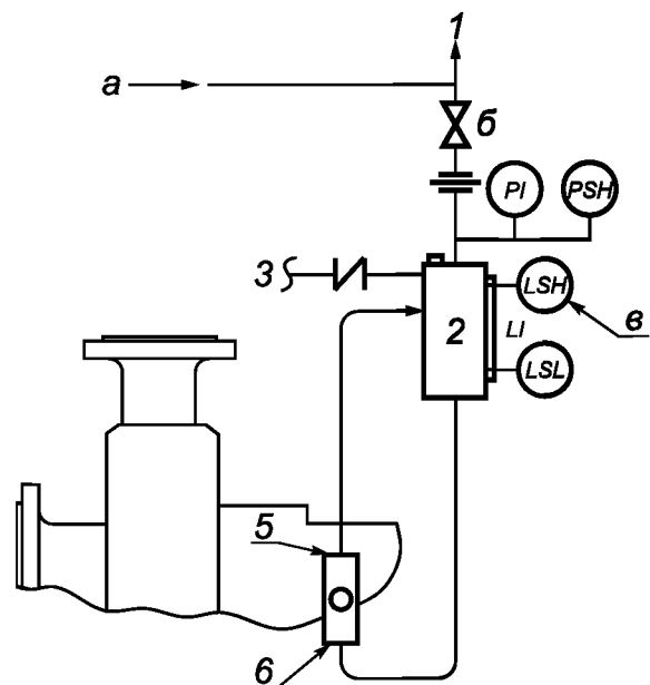
а) Трубопровод и схема измерительного прибора
