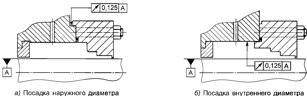
Рисунок 13 — Зарегистрированная соосность камеры уплотнения
