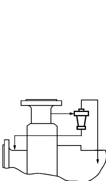
а) Трубопровод и схема измерительного прибора
