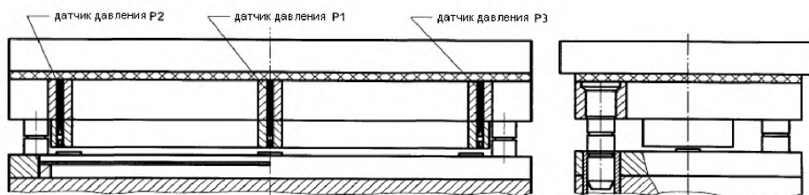
Рисунок 4 – Испытательная форма с датчиками
