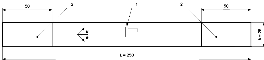
Рисунок 1 – Образец ламината с указанием ориентации армирующего наполнителя
