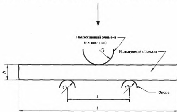
Рисунок 2 — Конфигурация нагружения
