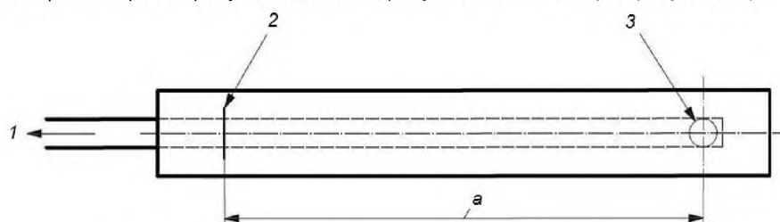
Рисунок А.1 – Оборудование для нарезания испытываемых проб длиной до 5 м
