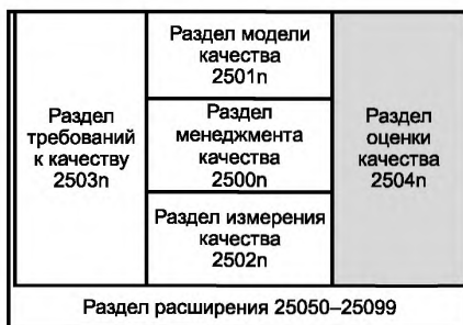
Рисунок 1 — Организация SQaRE серии международных стандартов
