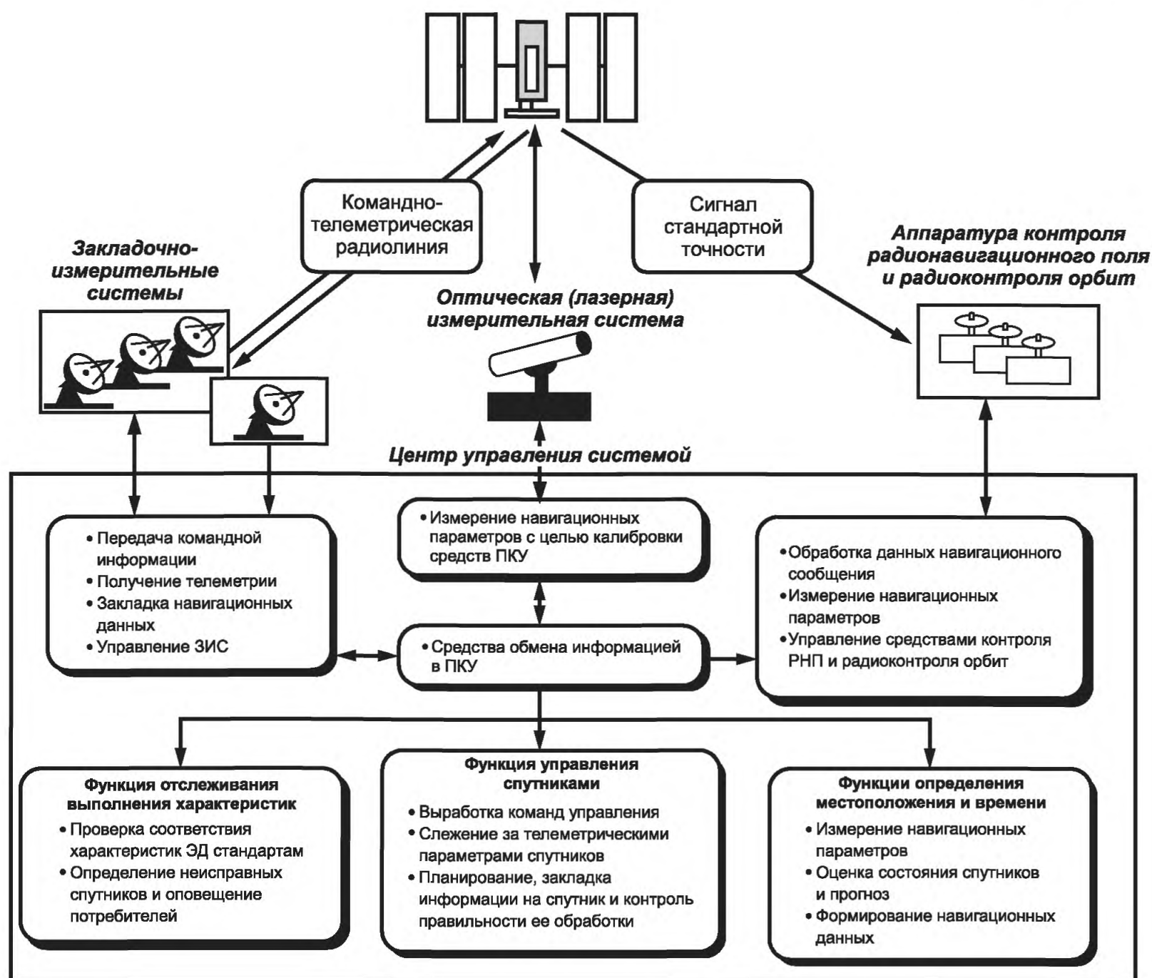
Рисунок А.2 — Процесс управления системой спутников
