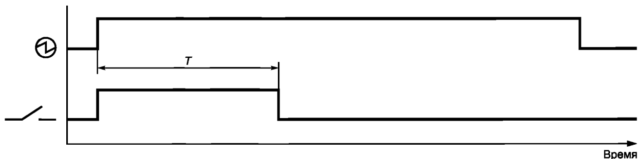
Рисунок 12 — Реле интервала
