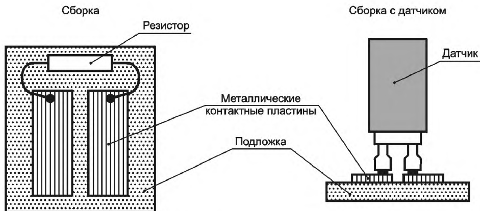
Рисунок 3 — Сборка для проверки сопротивления
