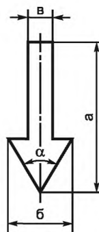
a = 180-200 \text{ мм} ; b = 80-100 \text{ мм} ; B = 30-40 \text{ мм} ; \alpha = 60^\circ-70^\circ
