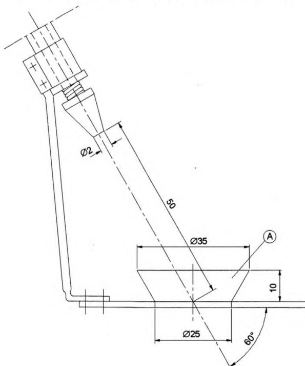
Рисунок 101 – Устройство для разбрызгивания
