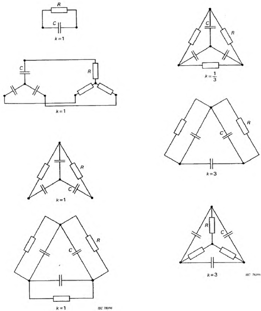
Рисунок В.1 — Значения k в зависимости от метода соединения резисторов с блоками конденсаторов
