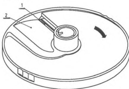
1 – режущий рабочий орган; 2 – наклонная пластина
