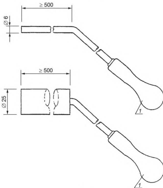
1 — ручка Рисунок А.1 — Конструкция щупов
