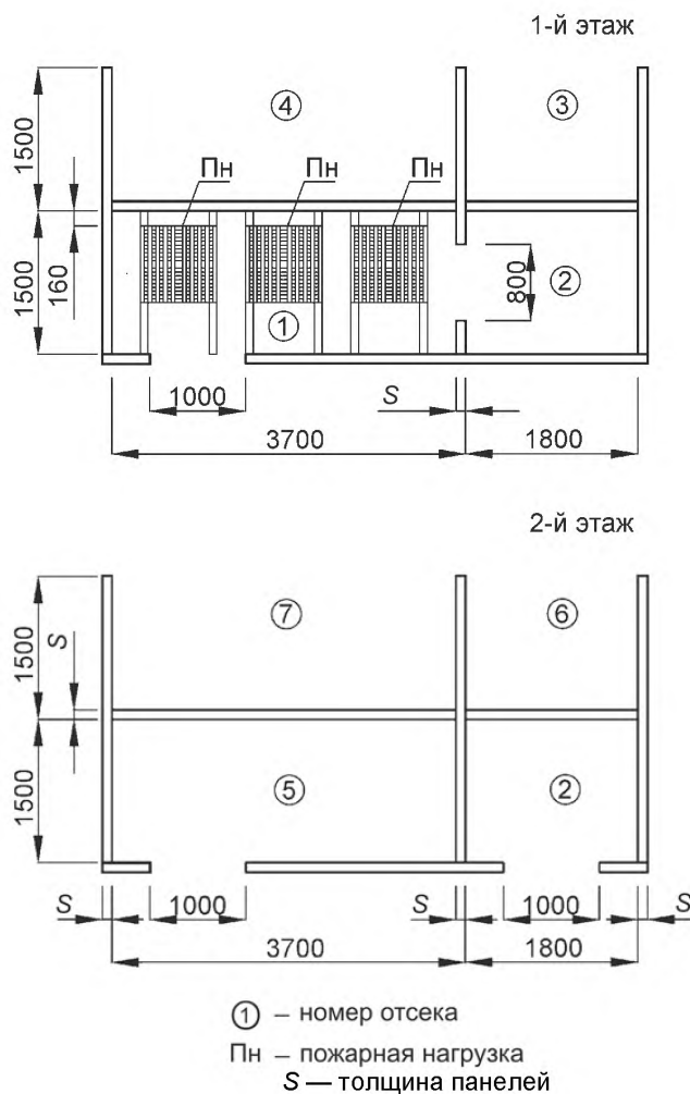
Рисунок Г.4 – Позэтажные планы
