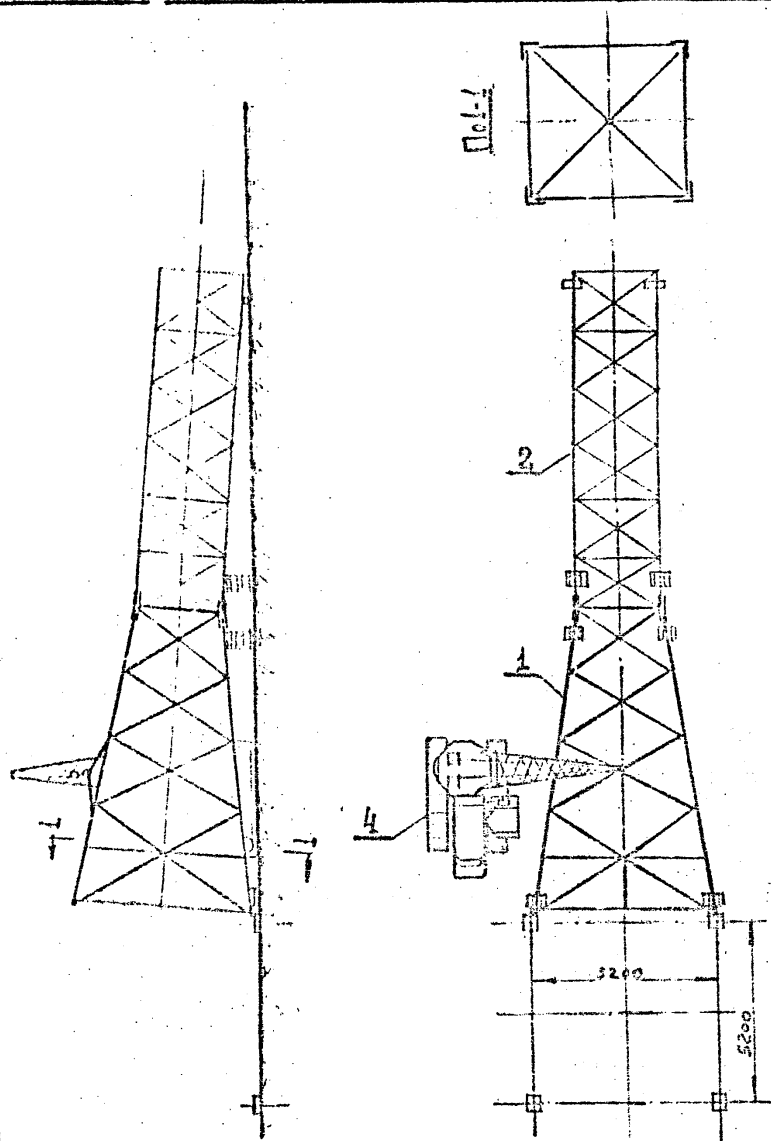
Рис. 33 Сборка 1-й секции ствола опоры У220-1
