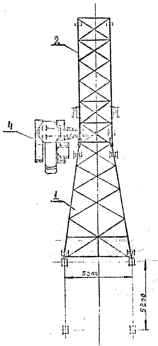
Рис. 32 Сборка 2 ой секции ствoла опоры У220-1
