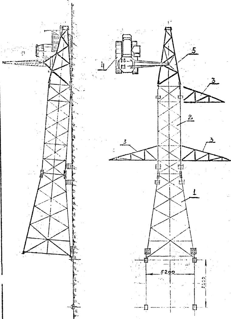
Рис. 34 Пристыковка тросов и тросостойки к стальной опоре 4220-1
