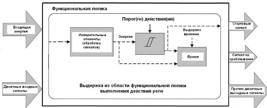
Рисунок 1 — Функциональный блок диаграмм выполнения защиты
