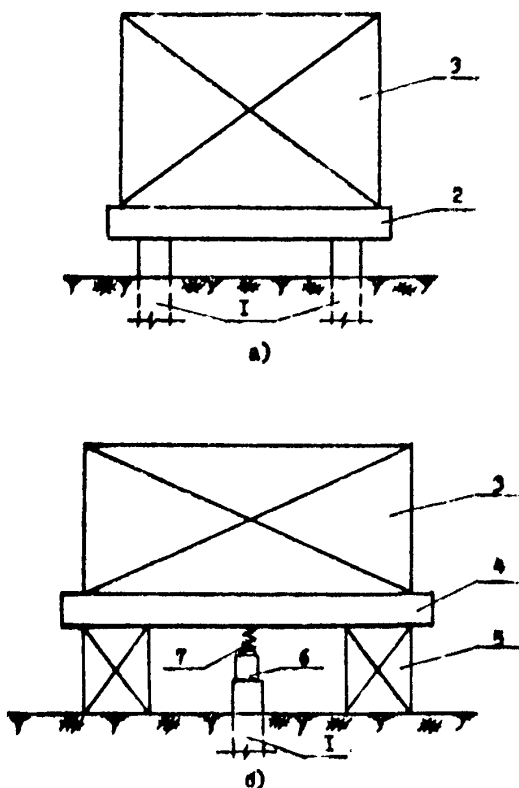
Рис. 2 Схемы загрузки поднимаемых конструкций при сезонных водонотных (1-пан; 2-ростерк; 3-груз; 4-загрузочная платформа; 5-опорная клетка; 6-домкрат; 7-пру- тинный вибростатор)
