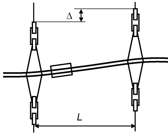
Рисунок 1 – Схемы к определению перегиба
