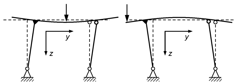
Рисунок 2 – Схемы деформаций металлической конструкции козлового крана
