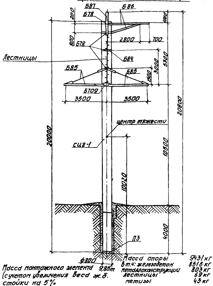
Рис. 0-3. Анкерно-угловая опора УБ220-7 (проект СЗО ЭСП 7275 тм-11)
