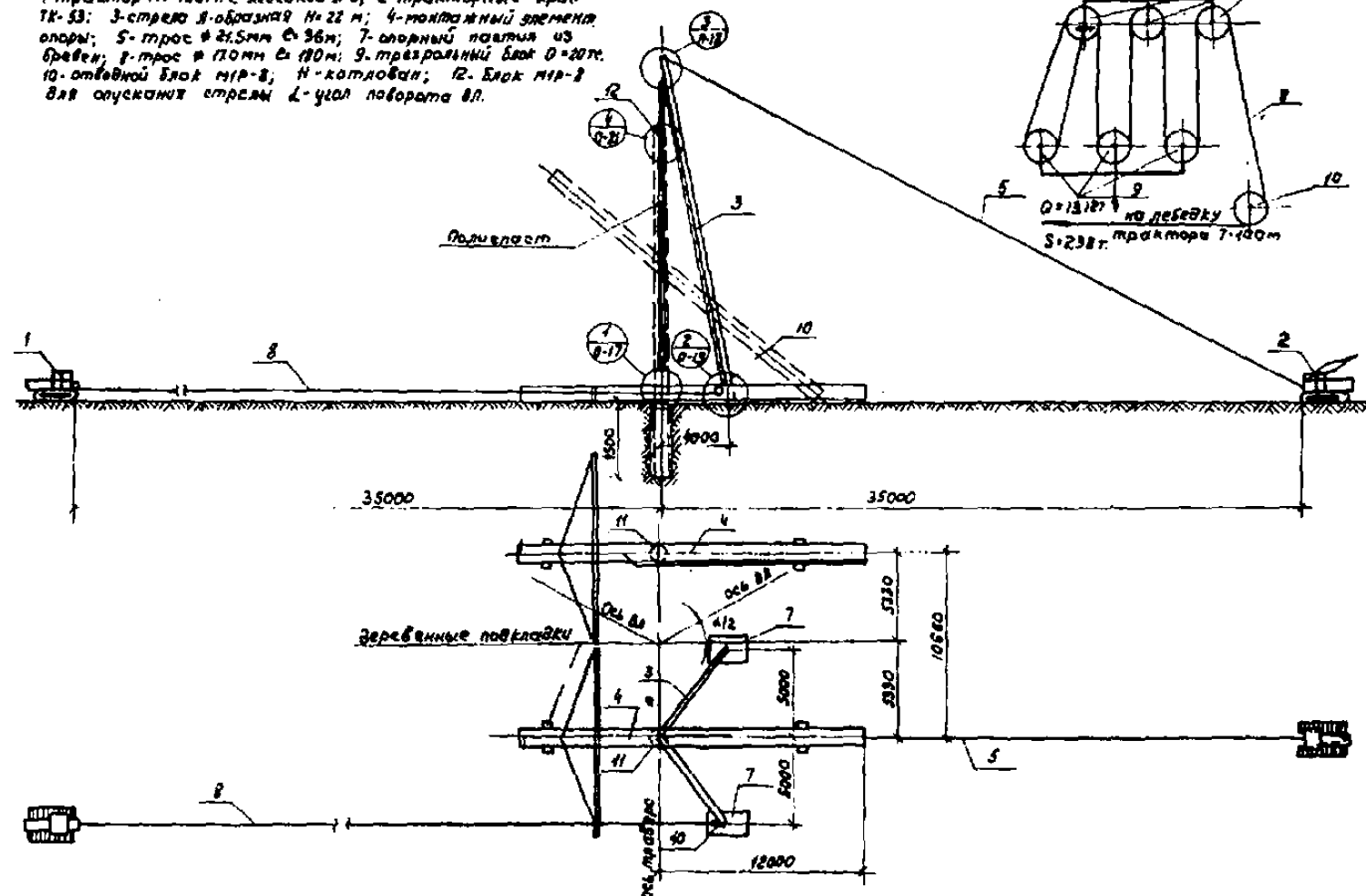
Рис. 14-1. Установка монтажных элементов опоры УБ 330-3 с помощью передвижной стрелы.
