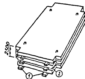
Панели перекрытий 1 - подкладки 150×100 мм 2 - прокладки 80×80 мм
