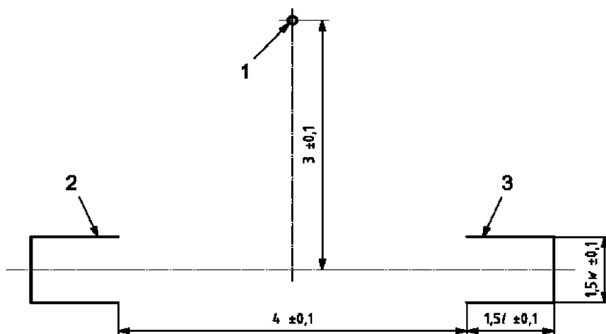
Рисунок 1 — Испытательная трасса
