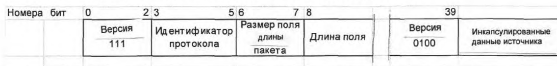
Рисунок 8 — Инкапсуляционный (вложенный) пакет
