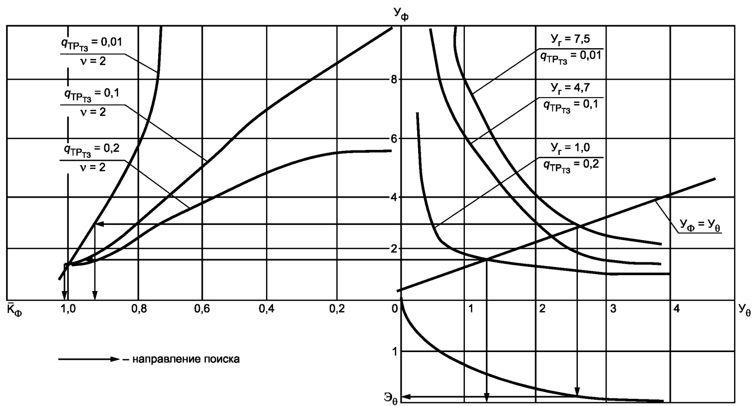
Рисунок 2 — Взаимосвязь между Y_\phi , Y_\theta , \bar{K}_\phi и эквивалентом наработки \Theta_\theta при Y_\phi = q_{TP_{T3}} \left( \frac{X_\theta}{X_\phi} \right)^v - 1 и Y_\theta = q_{TP_{T3}} \left( \frac{X_\phi}{X_\theta} \right)^v - 1
