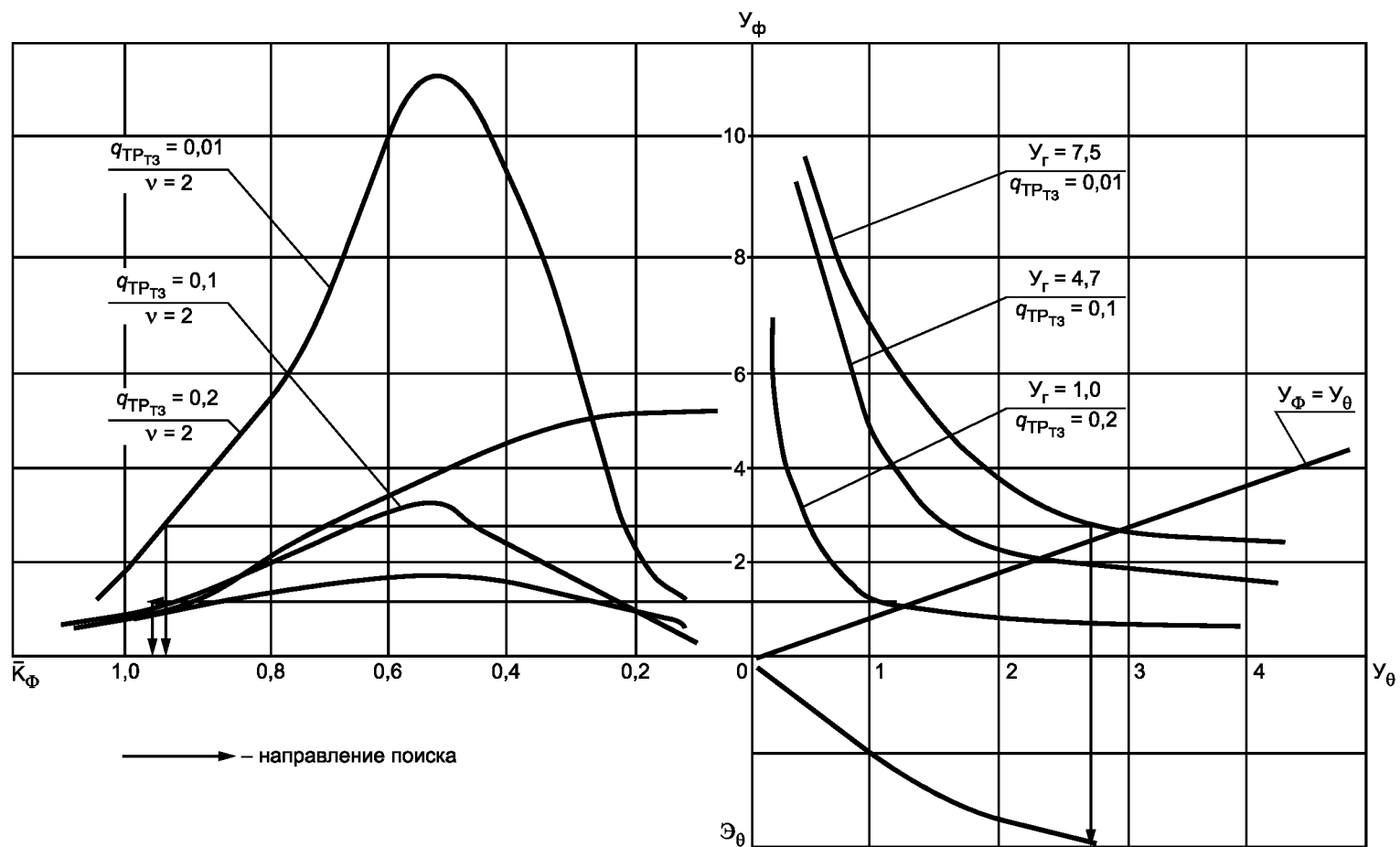
Рисунок 3 — Взаимосвязь между Y_\phi , Y_\theta , \bar{K}_\phi и эквивалентом наработки \Theta_\theta при Y_\phi = \frac{X_\phi^v + \frac{1}{X_\phi^v} - 1}{X_\theta^v + \frac{1}{X_\theta^v}} (v = 2)
