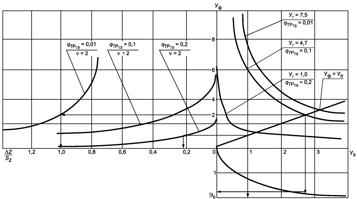
Рисунок 1 — Взаимосвязь между y_\phi , y_\theta , \frac{\Delta Z}{S_z} и эквивалентом наработки \Theta_\theta при y_\phi = \frac{1 - \Phi\left(\frac{\Delta Z}{S_z}\right)}{q_{TP13}}
