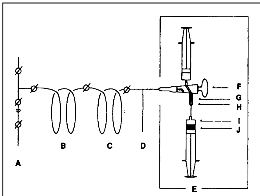
Рисунок А.1 — Лабораторная система для очистки двуокси углерода после завершения реакции изотопного обмена
