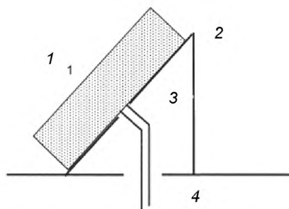
1 – солнечная система БГВ; 2 – пристройка к крыше; 3 – температура внутри помещения; 4 – трубы системы, через отверстие в крыше
