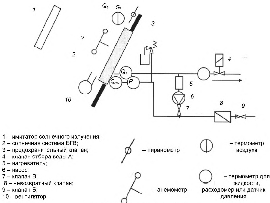
Рисунок В.6 – Схема структуры испытания
