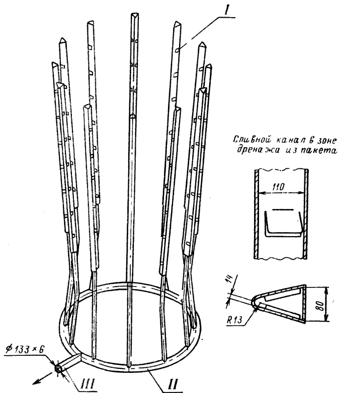
I — вход воды, отсепарированной в жалюзийных пакетах; II — коллектор отсепарированной воды; III — выход воды
