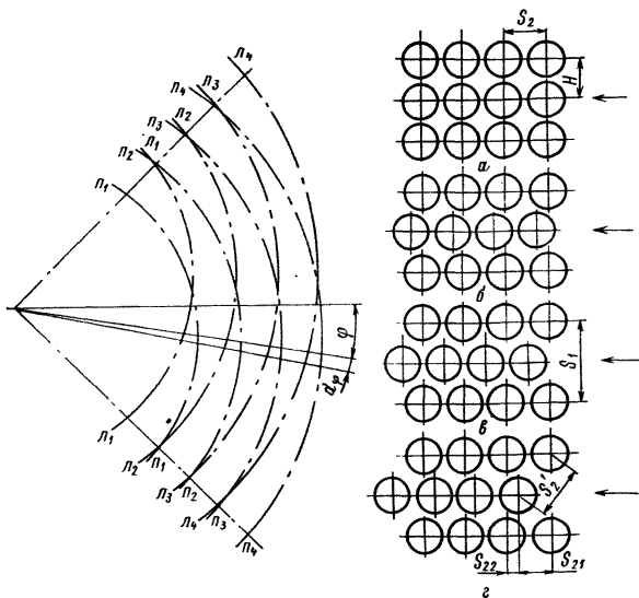
а — \varphi = 0; 45^\circ ; б — \varphi = 12^\circ ; в — \varphi = 22,5^\circ ; г — \varphi = 33^\circ ; л 1 , л 2 , л 3 , л 4 — левая навивка; п 1 , п 2 , п 3 , п 4 — правая навивка
