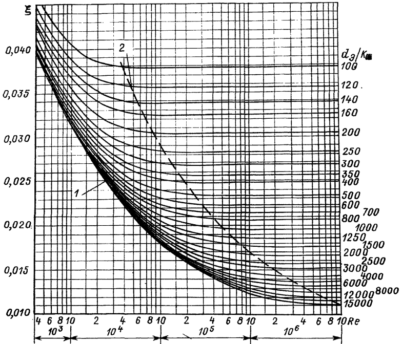
1 — гладкие трубы; 2 — Re_{кр} — предельные значения чисел Рейнольдса (справа от кривой 2 находится область квадратичного закона сопротивления);
