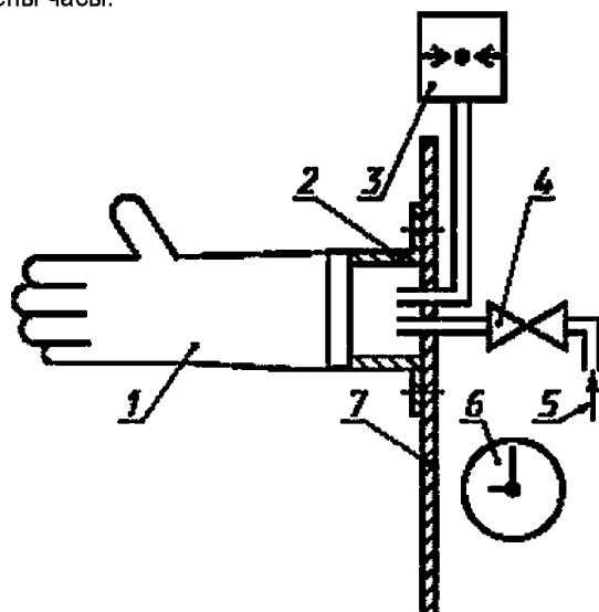
1 — насадка для крепления перчатки; 2 — испытываемая перчатка; 3 — вертикальная плита; 4 — манометр; 5 — клапан наполнения; 6 — сжатый воздух; 7 — часы
