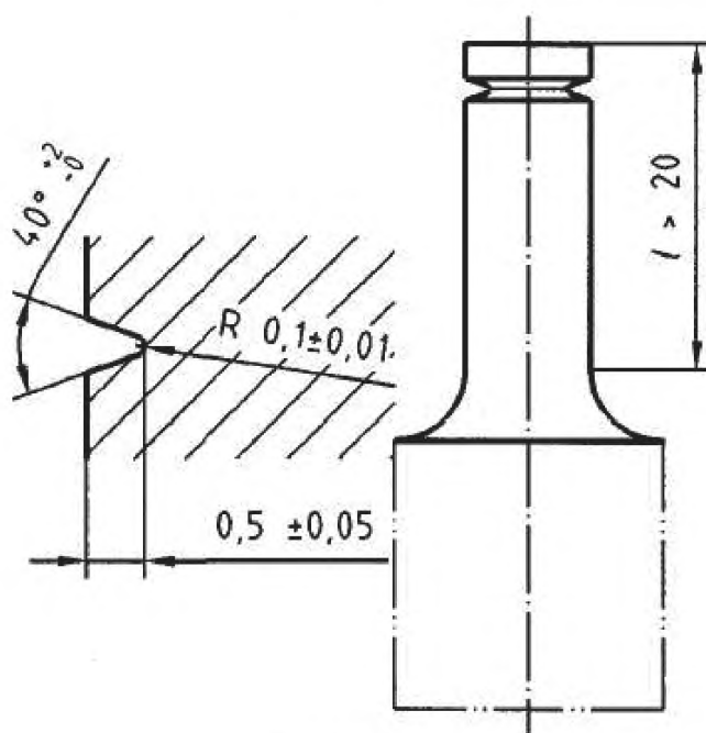
Рисунок 3 — Имплант кольцевой
