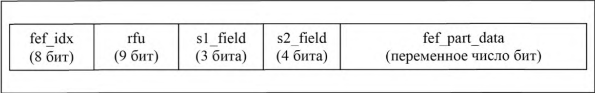
Рисунок 12 — Блок FEF с I/Q-данными как полезная нагрузка
