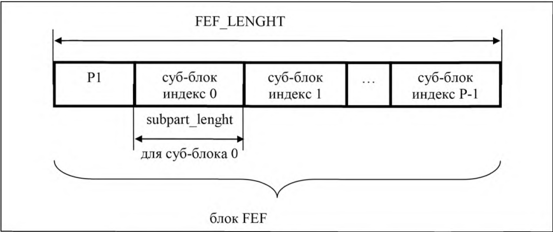
Рисунок 13 — Деление блока FEF на суб-блоки
