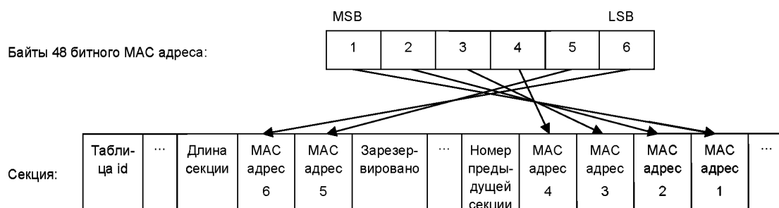
Р и с у н о к 4 — Отображение байтов MAC адреса в полях секции
