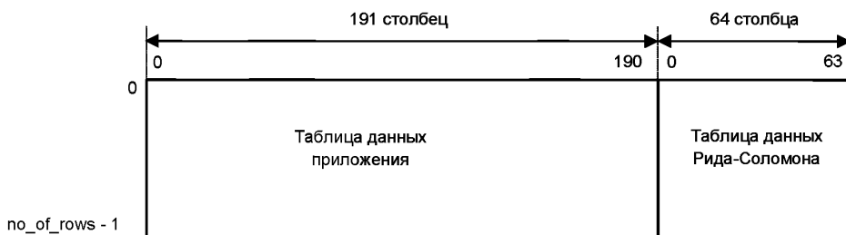
Р и с у н о к 8 — Структура кадра MPE-FEC
