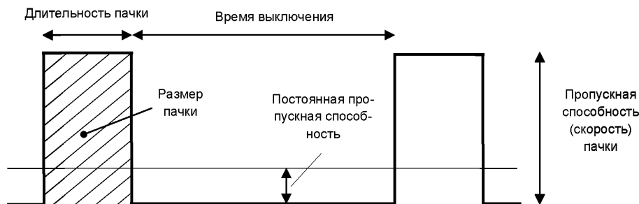
Р и с у н о к 6 — Основные параметры пачки
