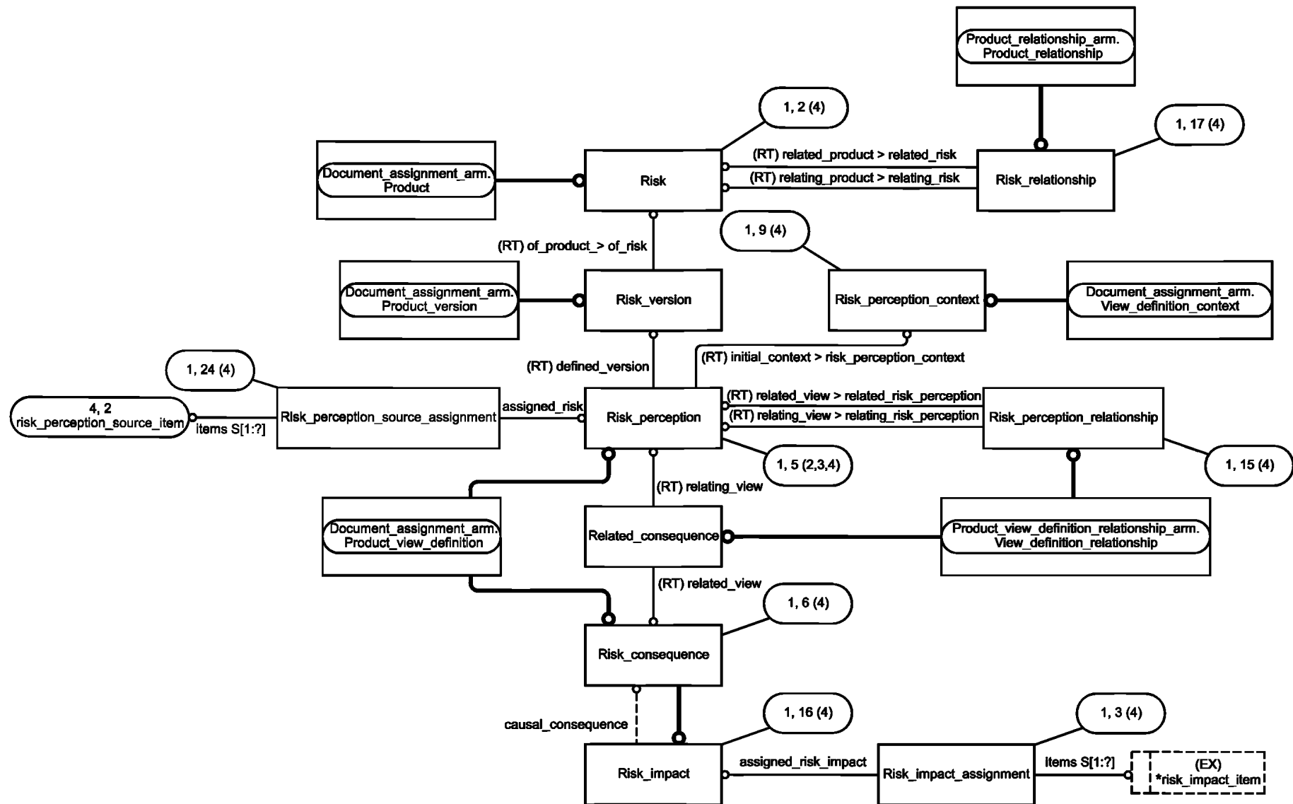
Рисунок С.2 — Представление ПЭМ на уровне объектов в формате EXPRESS-G (диаграмма 1 из 4)
