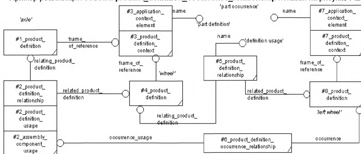
Рисунок F.2 – Пример реализации объекта product_definition_occurrence_relationship
