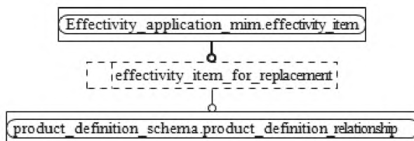
Рисунок D.2 – Представление ИММ на уровне объектов в формате EXPRESS-G (диаграмма 1 из 1)
