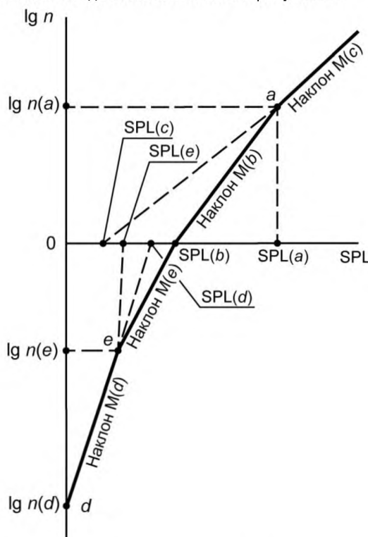
Рисунок Г.1 — График зависимости логарифма воспринимаемой шумности от уровня звукового давления в третьоктавной полосе
