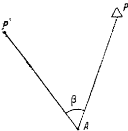
Рис. 1. Отыскание центра пункта по одному ориентирному пункту
