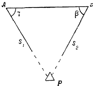
Рис. 3. Отыскание центра пункта по двум ориентирным пунктам
