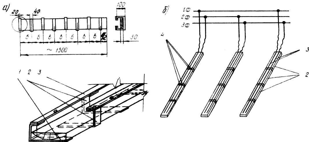
Рис. II. Накладной щит с полосовыми электродами (а) и схема коммутации электродов (б) при электропрогреве стыков между плоскими плитами покрытия:
