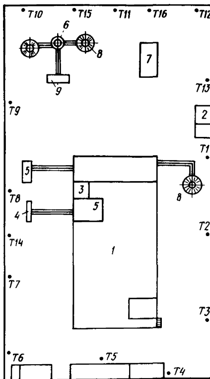
СХЕМА ГЕНЕРАЛЬНОГО ПЛАНА ГОРОДСКОГО МОЛОЧНОГО ЗАВОДА 1 – главный корпус; 2 – проходная; 3 – трансформаторная подстанция; 4 – градирня; 5 – компрессорная; 6 – камера переключения; 7 – котельная; 8 – резервуар; 9 – насосная станция
