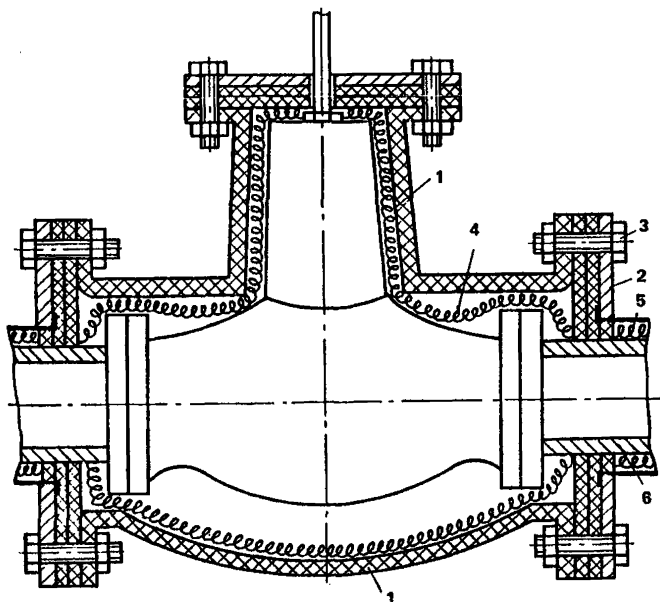
Рис. 14. Звукоизоляция небольшого вентиля
