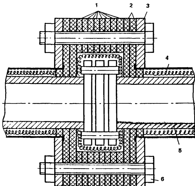
Рис. 12. Звукоизоляция фланцевого соединения трубопровода 1 – войлочное кольцо; 2 – войлочный диск; 3 – прижимный диск; 4 – звукоизолирующий материал; 5 – трубопровод; 6 – стяжной болт
