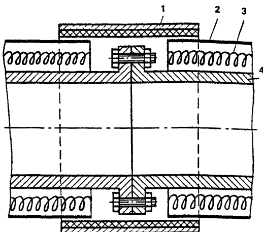
Рис. 13. Звукоизоляция фланцевых соединений трубопроводов небольших диаметров
